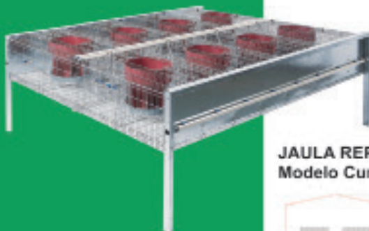
JAULA POLIVALENTE Modelo Euro-7 H-G/Grande
